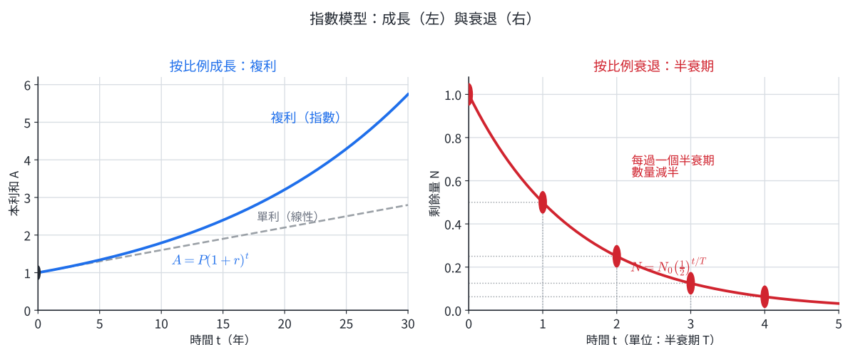
圖 2-3：指數模型。左——複利（指數，曲線）期數一大就遠遠把單利（線性，直線）甩開；右——半衰期衰退，每過一個半衰期 T 數量減半。
