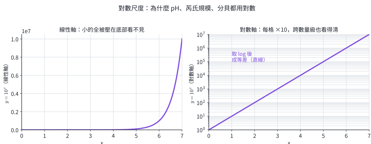
圖 2-4：同一條 y = 10^x 。左——線性軸上小值全被壓在底部看不見；右——改用對數軸，每格 \times 10 ，跨數量級也看得清，且取 \log 後成等差(直線)。
